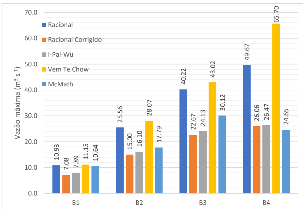
Figura 2. Vazão máxima para período de retorno de 25 anos.
