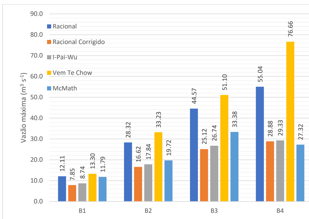
Figura 3. Vazão máxima para período de retorno de 50 anos.
