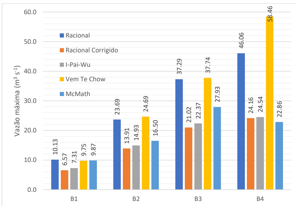
Figuras 1. Vazão máxima para período de retorno de 15 anos.
