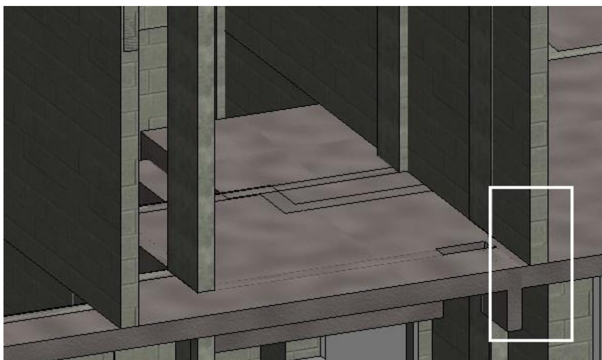
Figura 17 – Parede apoiando em laje sem viga
