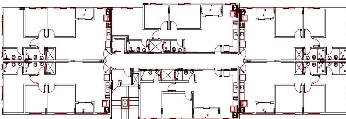
Figura 2 – Planta Baixa Pavimento Tipo
