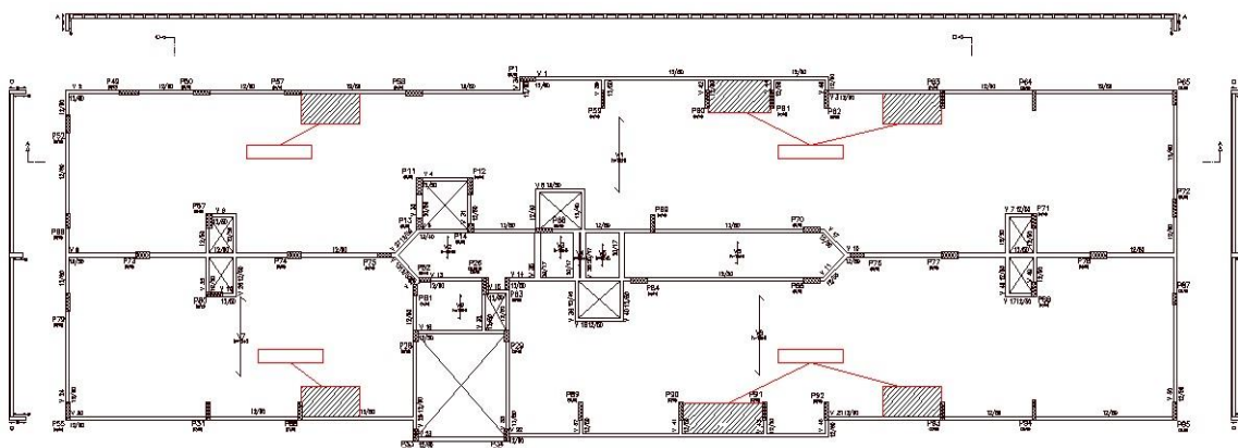
Figura 4 – Projeto de Forma Pavimento Tipo
