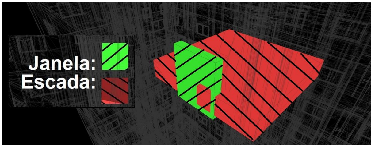
Figura 15 – Interferência entre janela e escada do pavimento térreo detectada no teste 4
