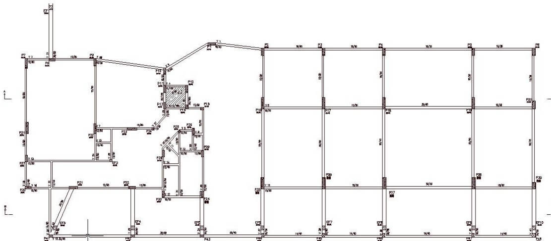
Figura 3 – Projeto de Forma Pavimento Térreo
