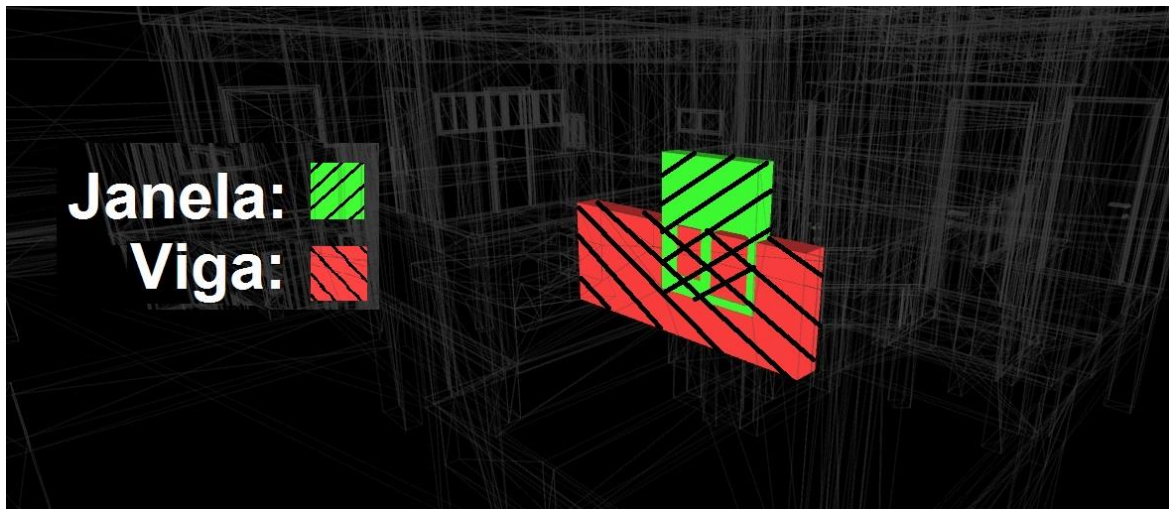
Figura 14 – Interferência entre janela e escada do 6º pavimento detectada no teste 4
