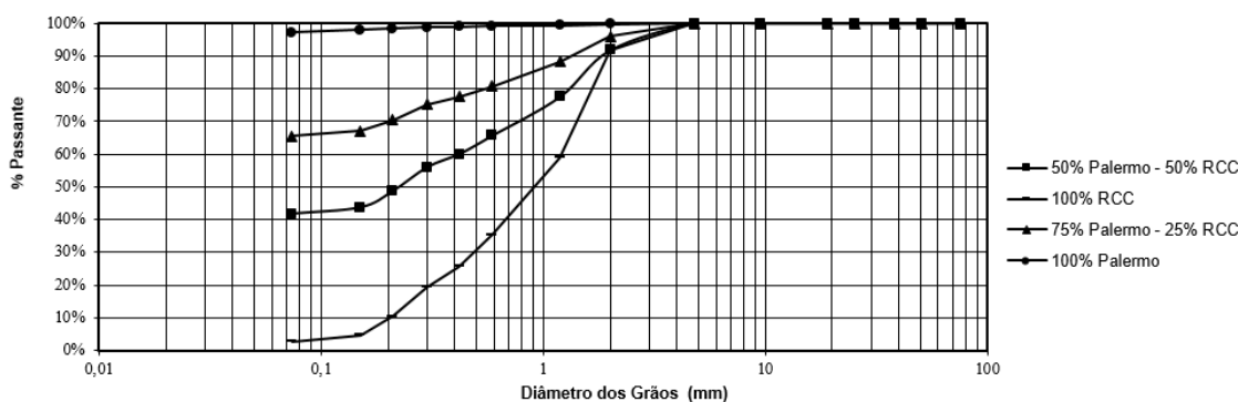
Figura 4. Curvas de distribuição granulométrica
