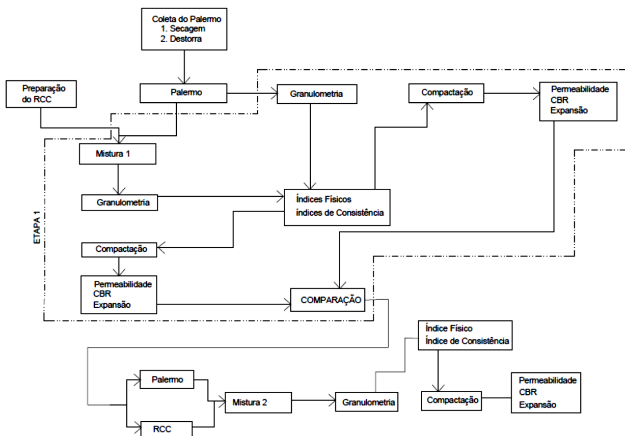
Figura 3. Fluxograma dos procedimentos descritos na metodologia do trabalho
